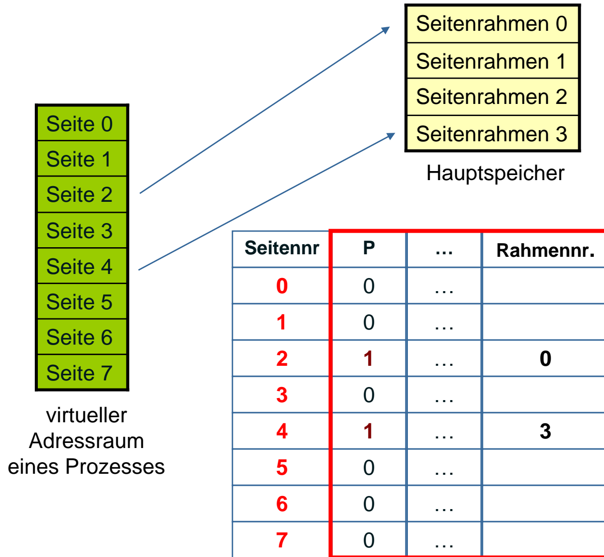
Seitentabelle des Prozesses im Hauptspeicher
